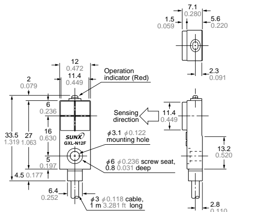
GXL-N12F type Sensor
